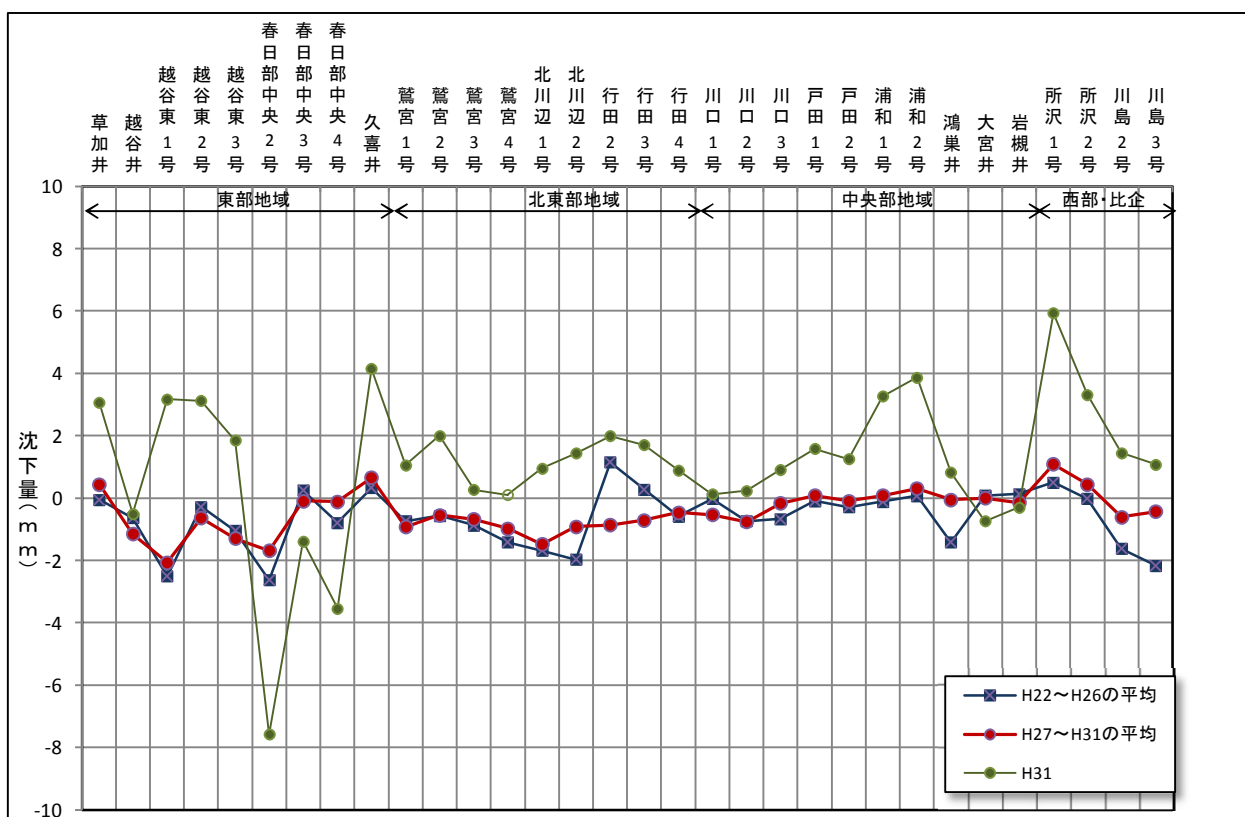
図2-10 平成22～26年・平成27年～31年(令和元年)の平均地盤変動量
