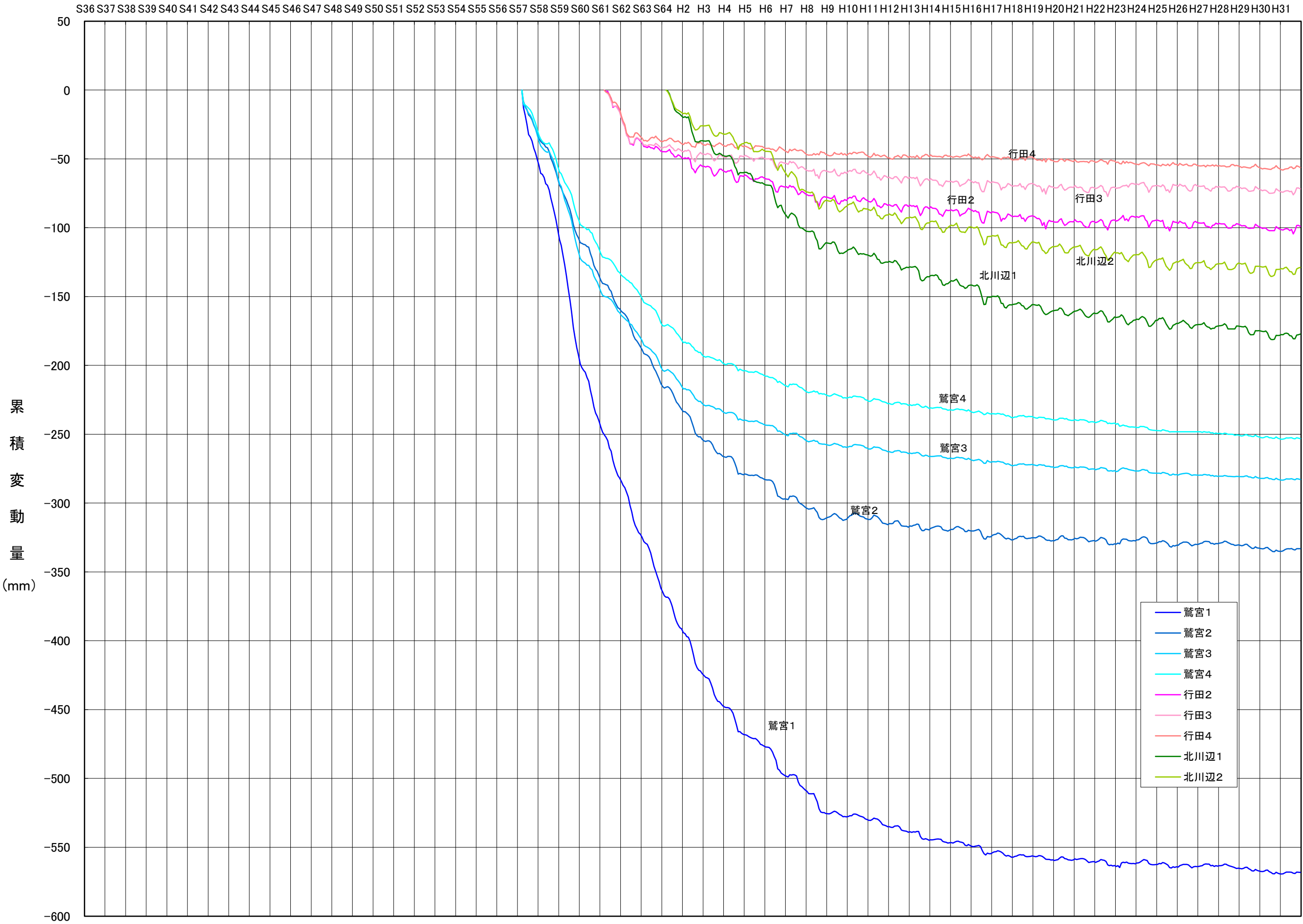
図 2-27 地盤変動経年変化(鷺宮, 行田, 北川辺)
