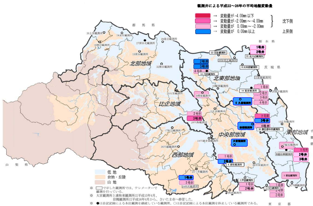
図 2-12 平成 22～26 年の平均地盤変動量 (基図は国土地理院基盤地図情報 25,000 を用いた。) 地形区分は、埼玉県地理環境情報 WebGIS 内のシェープファイル「表層地層分類」を加工して作成した。
