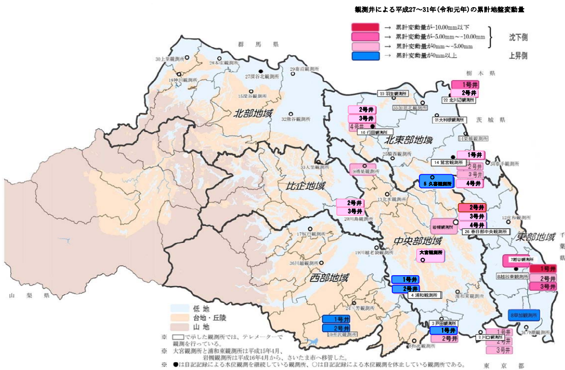
図 2-15 平成 27～31 年(令和元年)の累計地盤変動量
