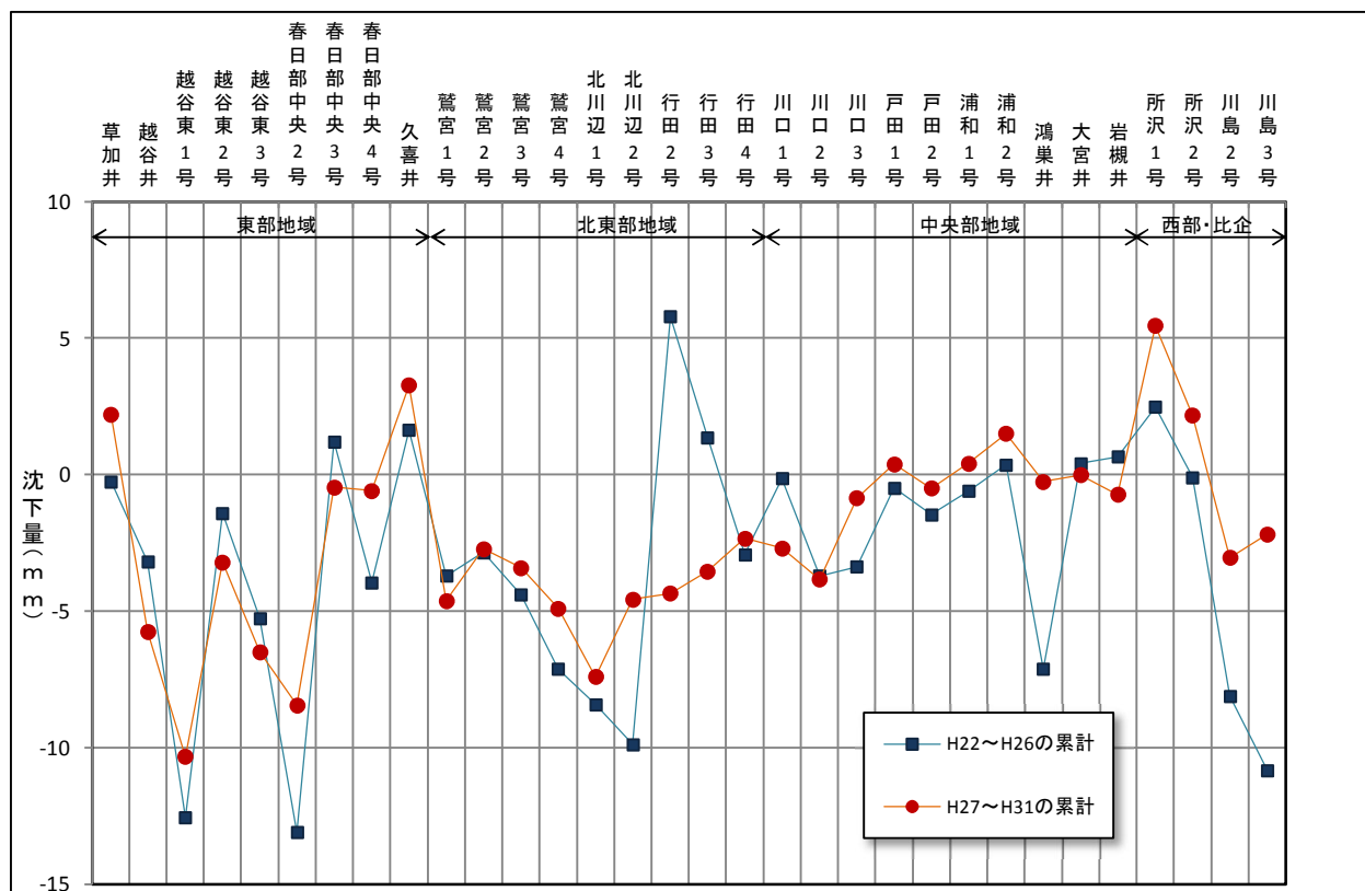
図2-11 平成22～26年・平成27年～31年(令和元年)の累計地盤変動量
